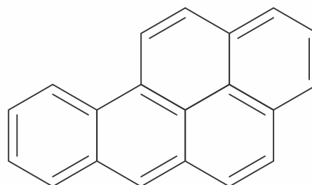
Benzopireno
