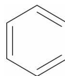
Benzeno
