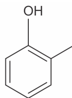
ortocresol
